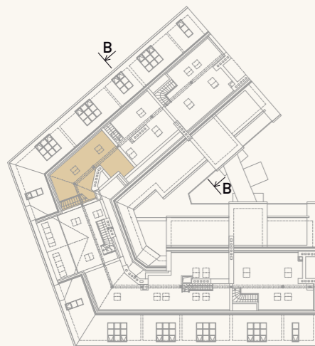
půdorys galerie
